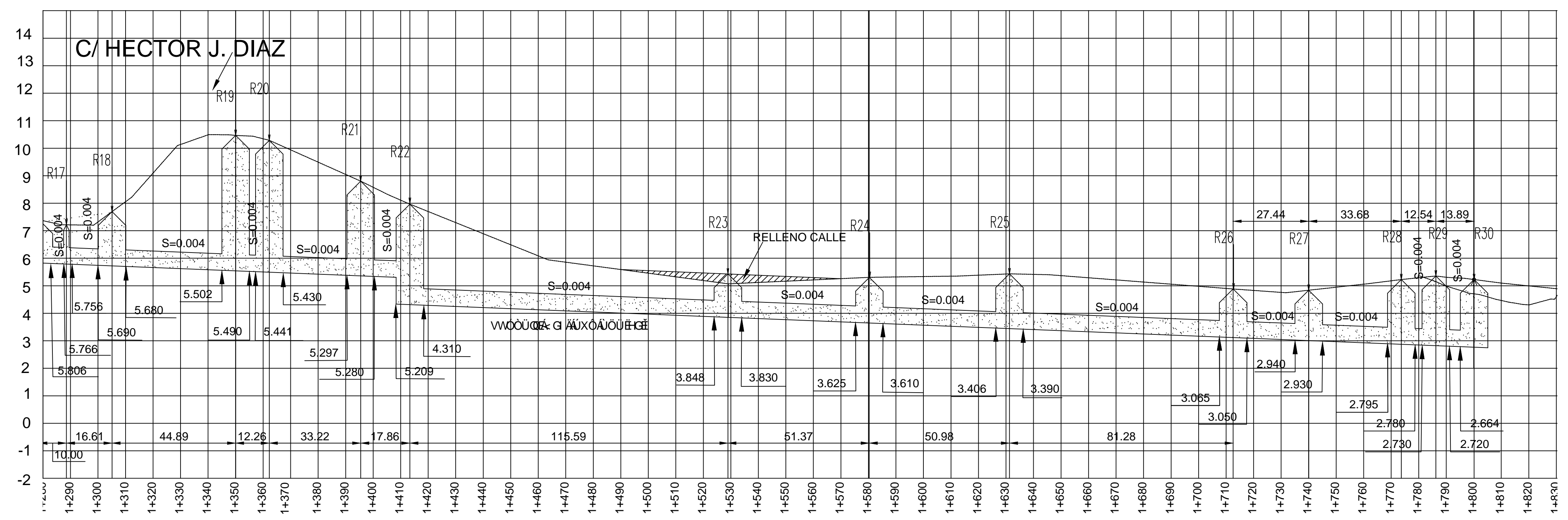
PERFIL C/HECTOR J. DIAZ ESC. 1:100/1:1000
